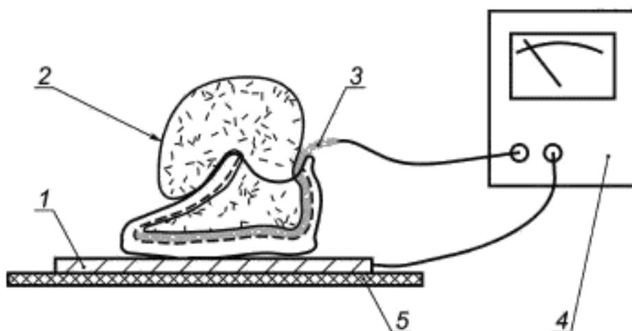
1 — пластина из нержавеющей стали (противозлектрод); 2 — наполненный металлическими деталями мешок; 3 — алюминиевая фольга (проводящий электрод); 4 — устройство измерения сопротивления, 5 — изолятор
